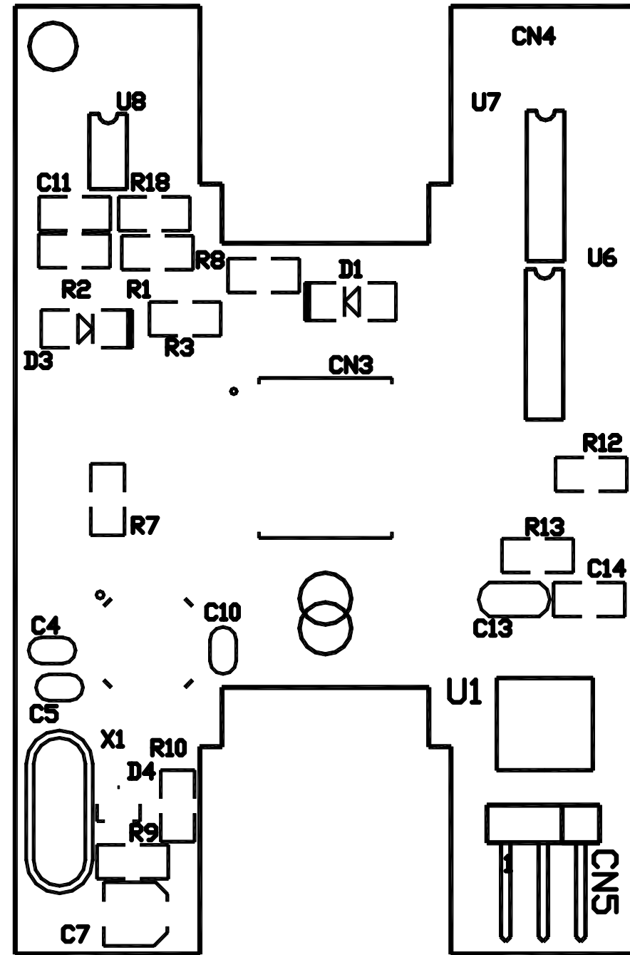
Bottom Overlay
