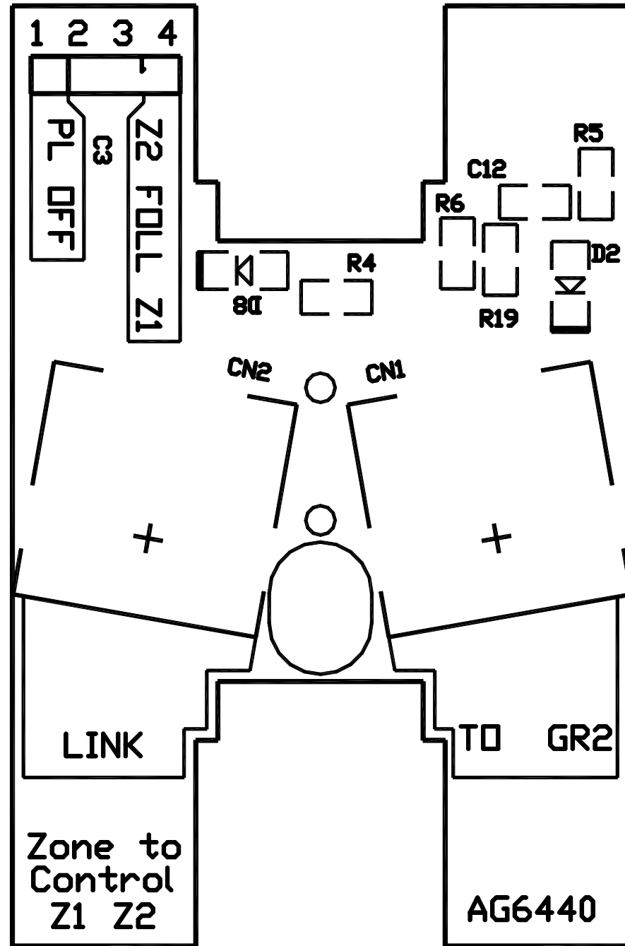
Top Overlay
