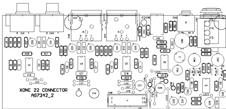
Connector 003-875
