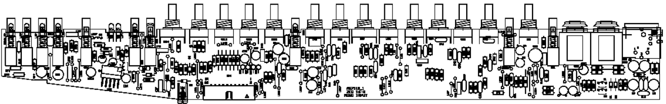
Mono i/p 003-817
