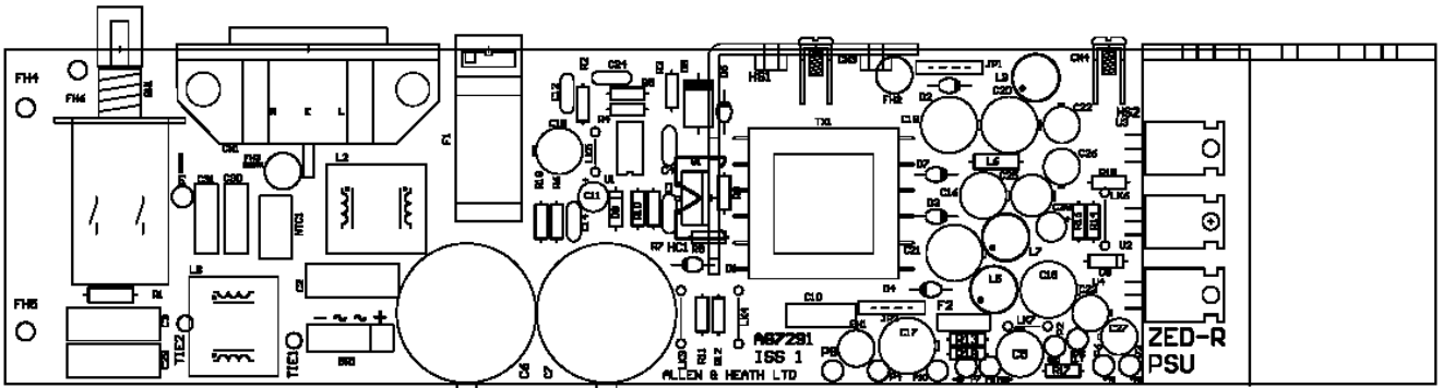
PSU 003-849
