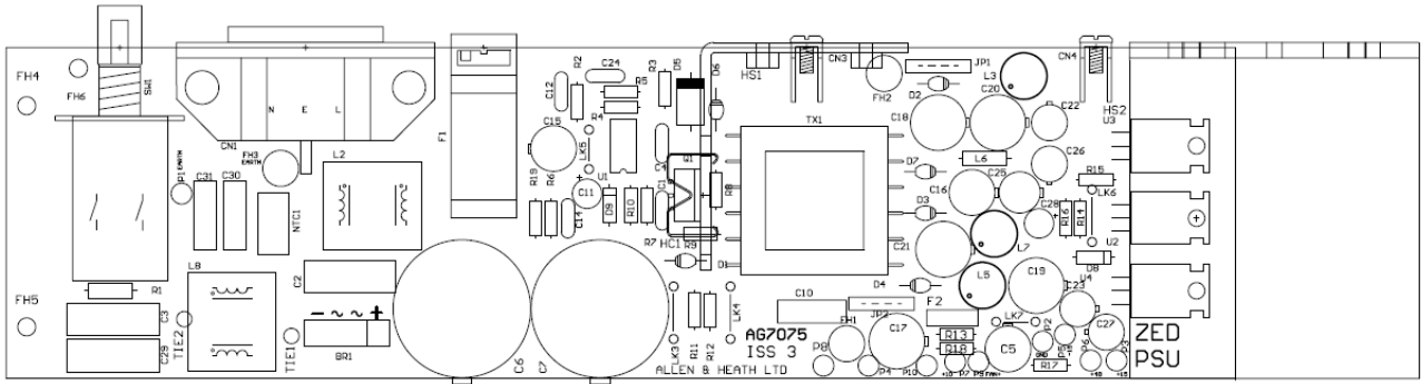
PSU 003-850
