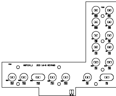
Keypad 003-826
