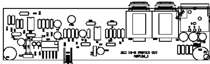
Master out 003-822
