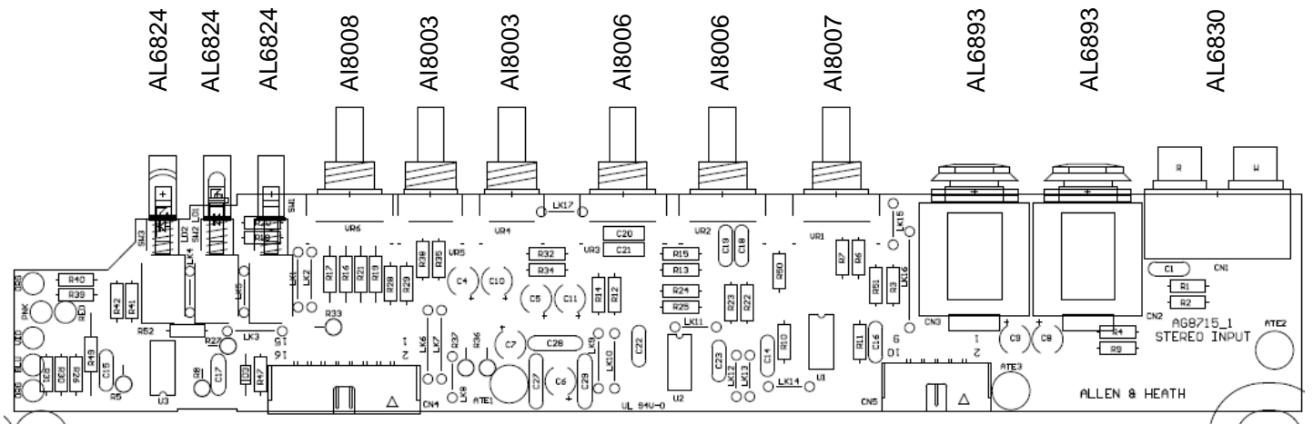
004-296 Stereo IP 1
