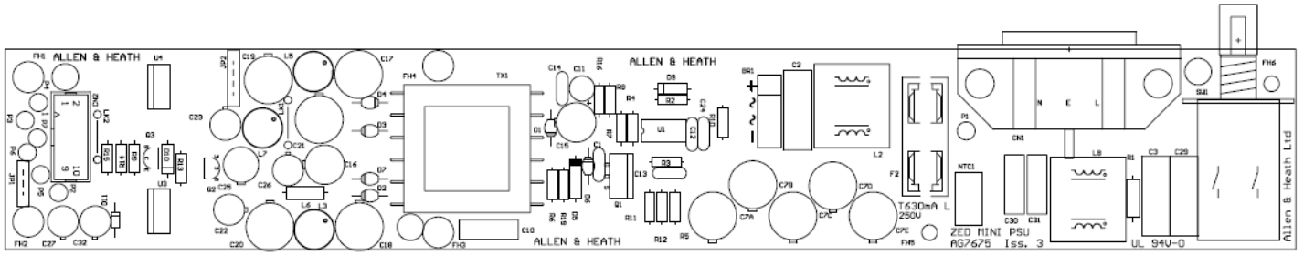
003-974 PSU
