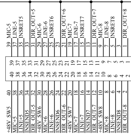
CN2 BOX 20X2 M 90 DEG
